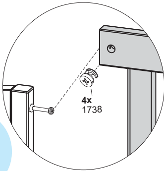
Detalhe E Detail E / Detalle E
