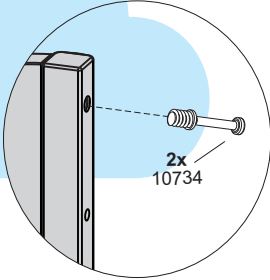
Detalhe C Detail C / Detalle C
