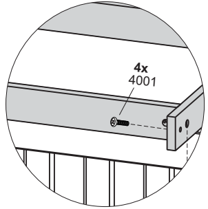
Detalhe G Detail G / Detalle G
