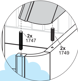
Detalhe F Detail F / Detalle F
